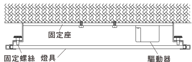
B. 安裝示意圖
